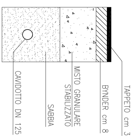
SEZIONE TIPO DI POSA CAVIDOTTO
