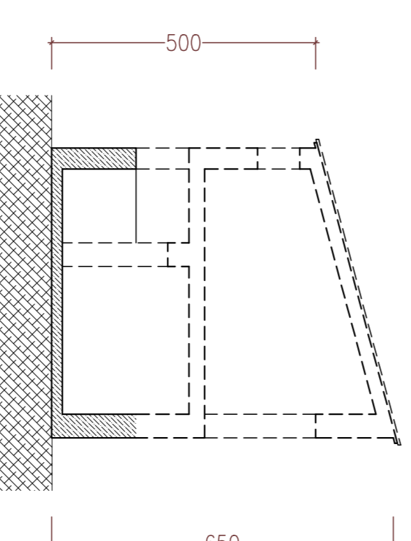
SEZIONE
