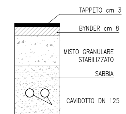
SEZIONE TIPO DI POSA CAVIDOTTO
