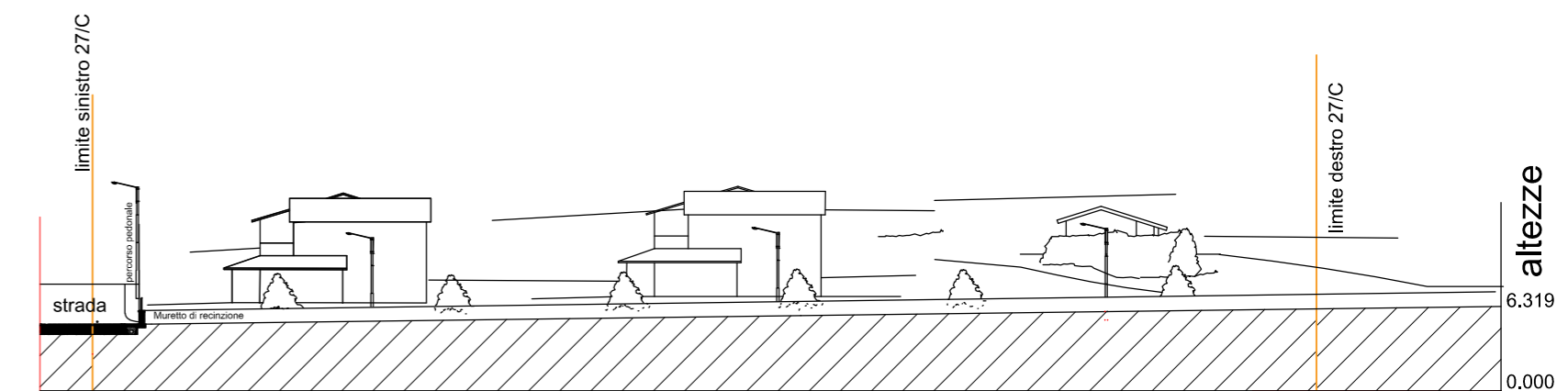
sez. C-C'
