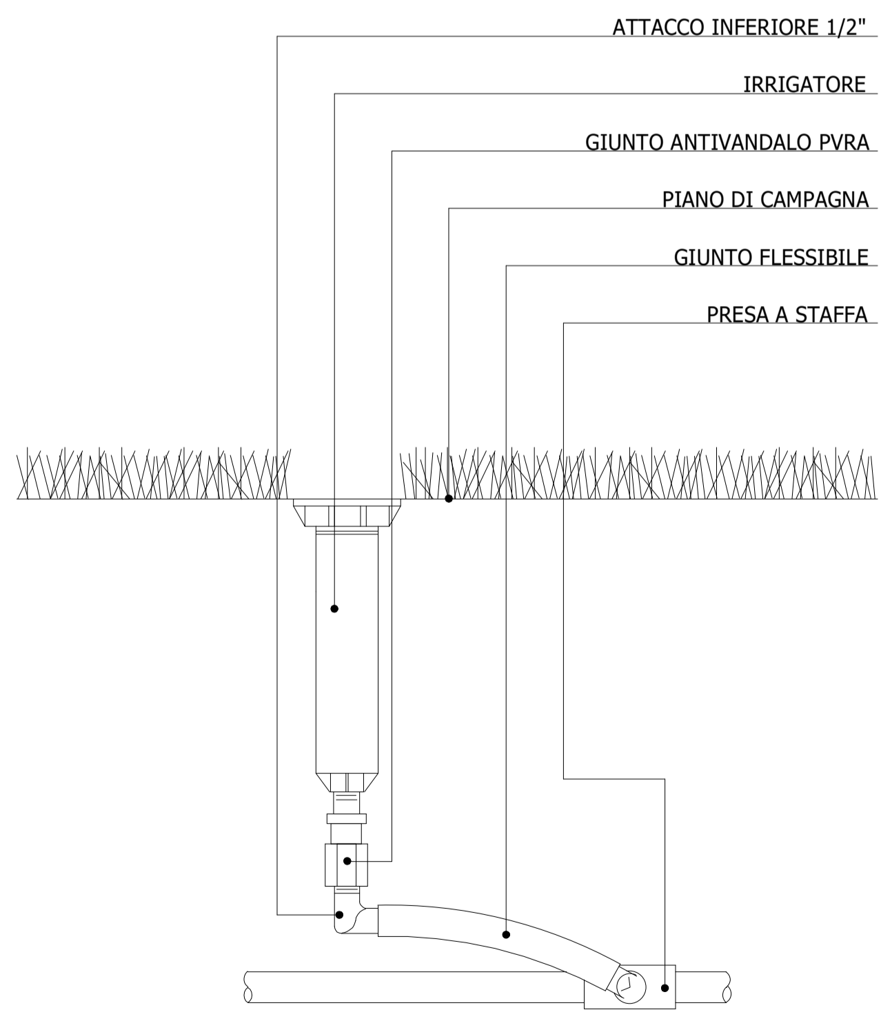
PARTICOLARE IRRIGATORE STATICO
