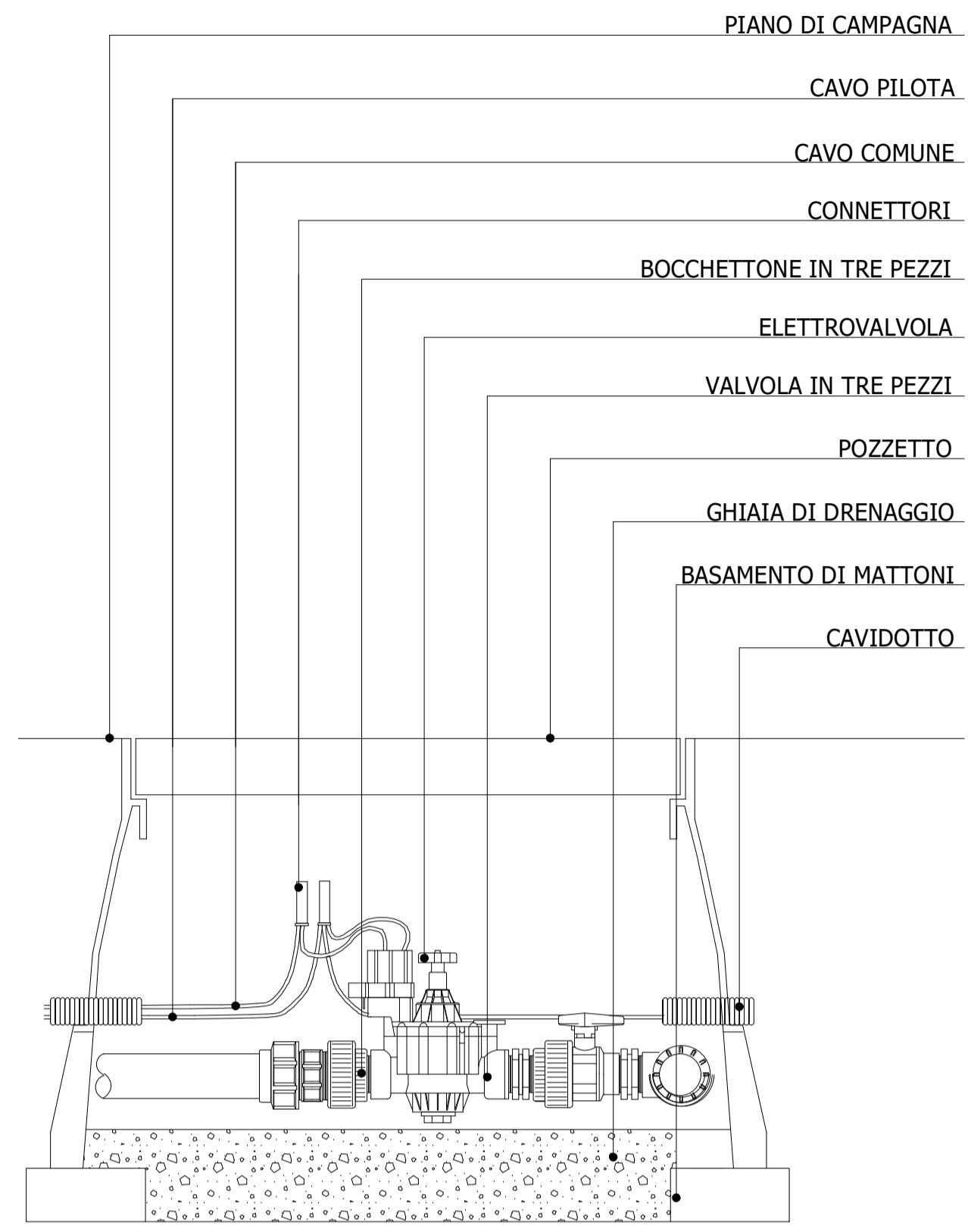
PARTICOLARE ELETTROVALVOLA
