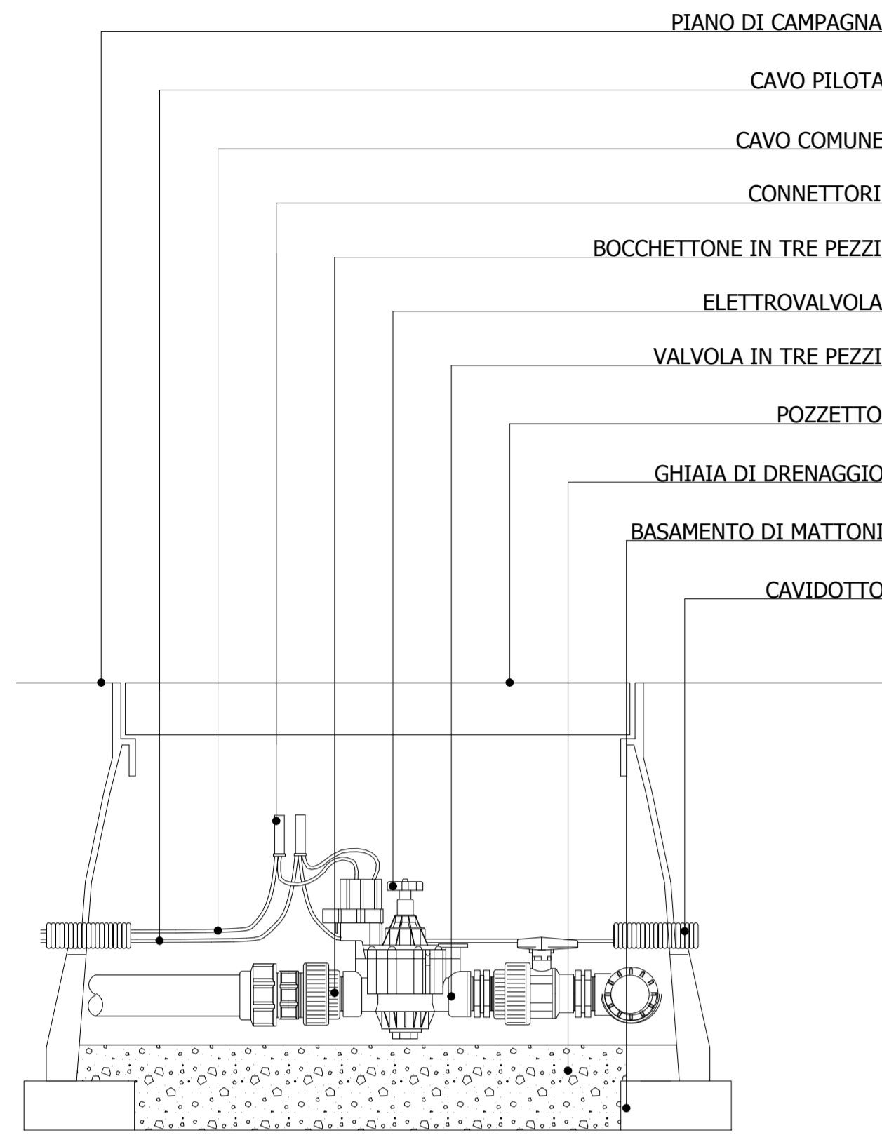
PARTICOLARE ELETTROVALVOLA
