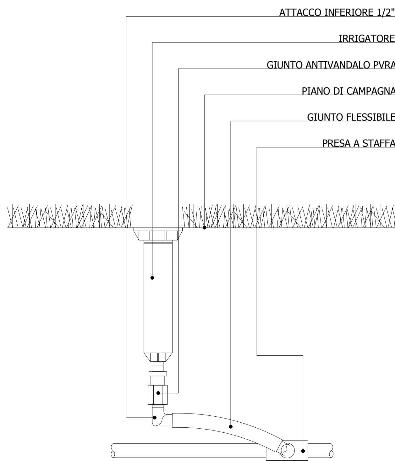
PARTICOLARE IRRIGATORE STATICO
